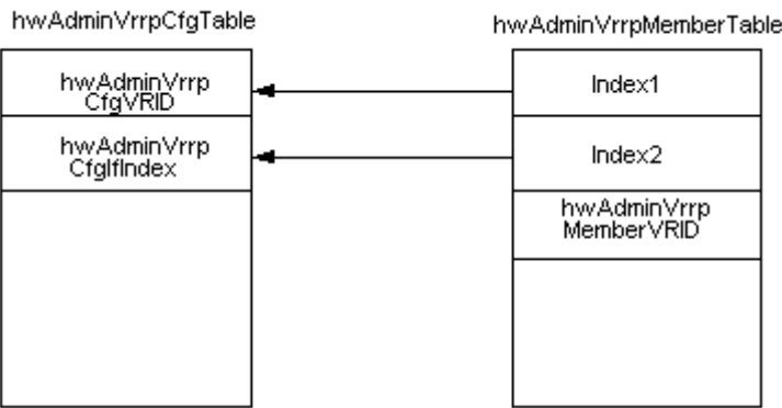
图 133-1 管理 VRRP 配置表和成员 VRRP 配置表的表间关系图
